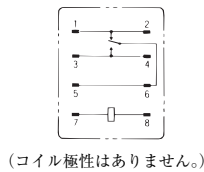
端子配置/内部接続図(BOTTOM VIEW) 形LY1 形LY1-D
