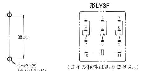
取り付け穴加工寸法 端子配置/内部接続図(BOTTOM VIEW)
