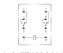
端子配置/内部接続図(BOTTOM VIEW) 形LY2(Z) 形LY2(Z)-D
