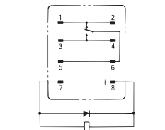
端子配置/内部接続図(BOTTOM VIEW) 形LY1 形LY1-D
