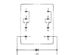
端子配置/内部接続図(BOTTOM VIEW) 形LY2(Z) 形LY2(Z)-D
