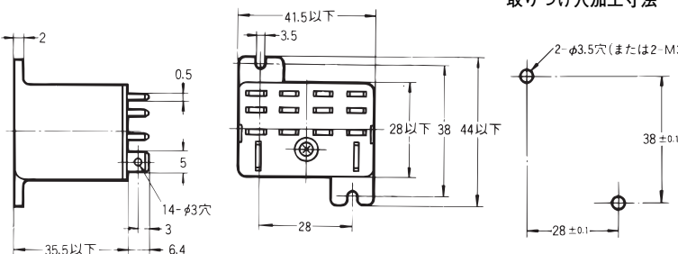
取り付け穴加工寸法 端子配置/内部接続図(BOTTOM VIEW)
