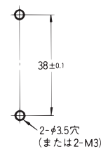
取り付け穴加工寸法
