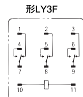
端子配置/内部接続図(BOTTOM VIEW)
