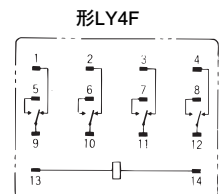
端子配置/内部接続図(BOTTOM VIEW)
