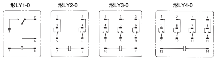
端子配置/内部接続図(BOTTOM VIEW)
