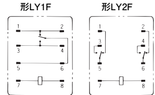
端子配置/内部接続図(BOTTOM VIEW)
