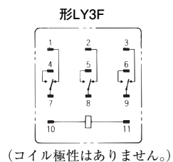
端子配置/内部接続図(BOTTOM VIEW)
