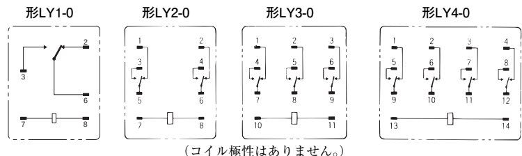
端子配置/内部接続図(BOTTOM VIEW)
