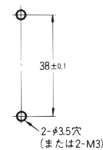
取り付け穴加工寸法
