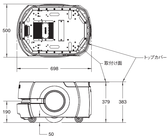
LD-60、LD-90、LD-90x、 LD-60 ESD、LD-90 ESD、LD-90x ESD
