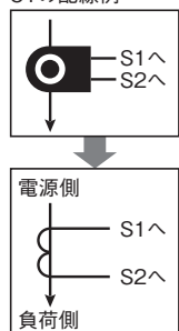
CTの配線例
