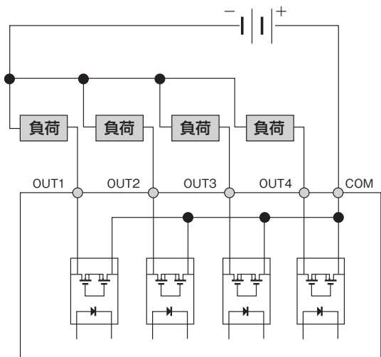
PNP出力接続図
