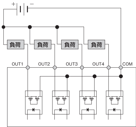
NPN出力接続図
