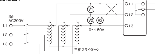
結線図1
