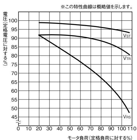
特性曲線(図)
