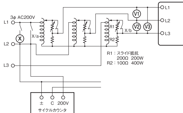
結線図2
