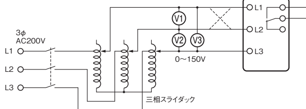
結線図1
