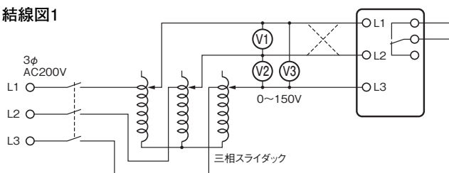
結線図1
