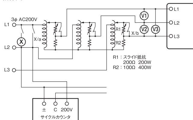
結線図
