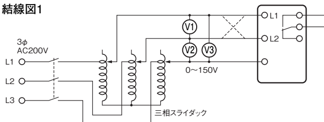
結線図1
