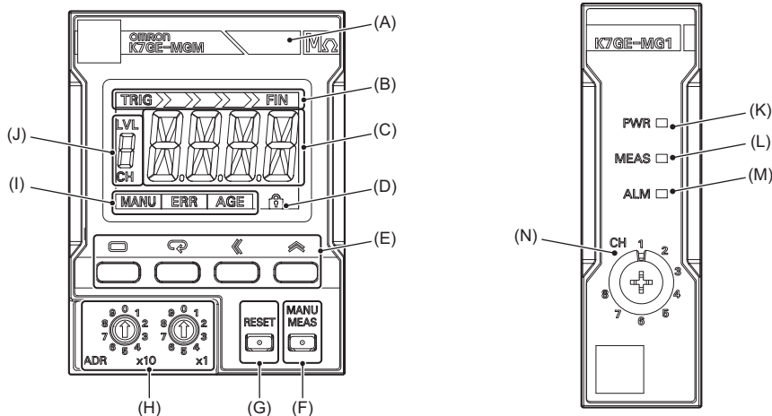
メインユニット 形K7GE-MGM
