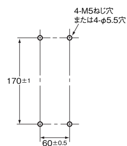
取り付け加工穴寸法
