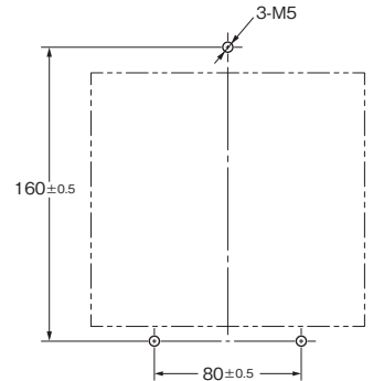
取り付け穴加工寸法
