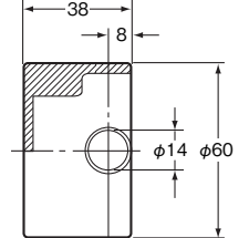
防じんキャップ寸法
