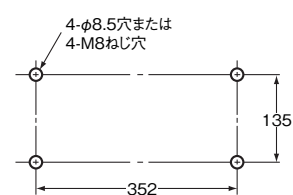
取り付け穴加工寸法
