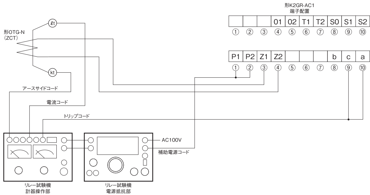
動作時間試験配線図 (形K2GR-AC1)
