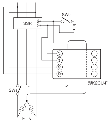
三相V結線の場合②
