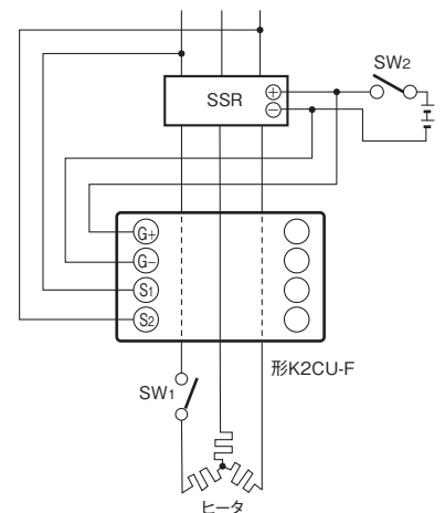
三相スター結線の場合
