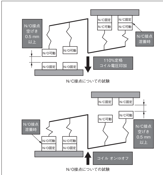
[リンクドコンタクトIEC60947-5-1]
