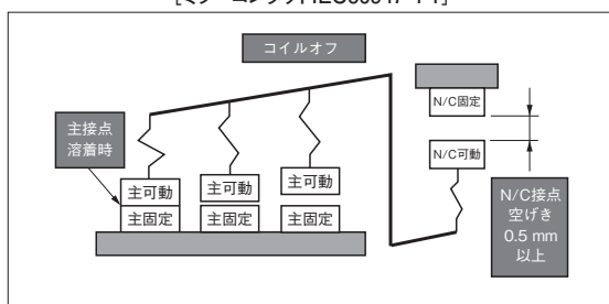
[ミラーコンタクトNEC60947-4-1]
