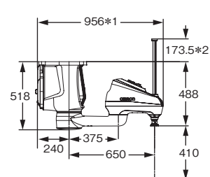
i4-650H 天吊りタイプ、ロングクイル
