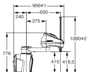
i4-650H、ロングクイル
