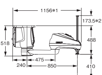
i4-850H 天吊りタイプ、ロングクイル
