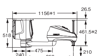
i4-850H 天吊りタイプ
