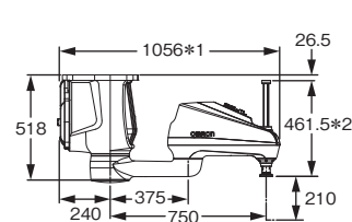
i4-750H 天吊りタイプ
