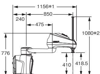
i4-850H、ロングクイル
