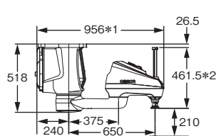
i4-650H 天吊りタイプ
