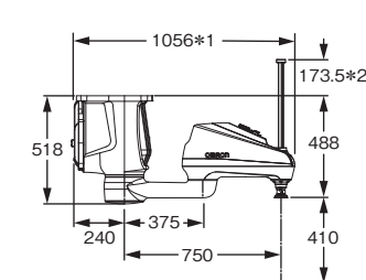
i4-750H 天吊りタイプ、ロングクイル
