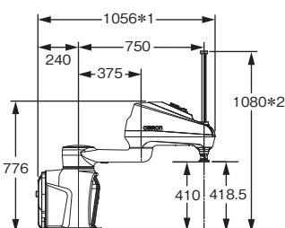
i4-750H、ロングクイル
