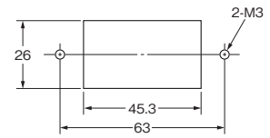
取り付け穴加工寸法
