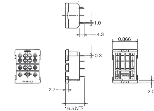
端子配置/内部接続図
