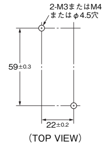
取り付け穴加工寸法
