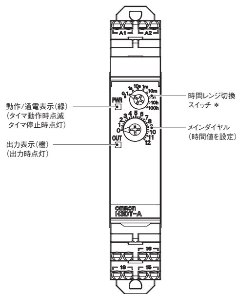
正面図
