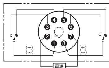
形H3CR-A8S (トランジスタ出力タイプ)
