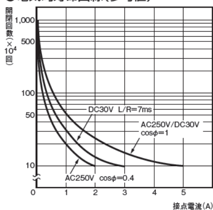
●電気的寿命曲線(参考値)
