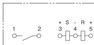
端子配置/内部接続図 (TOP VIEW)
