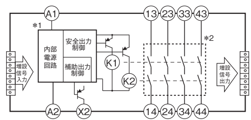
G9SX-EX401-□/G9SX-EX041-T-□ (増設ユニット/増設ユニットオフディレイタイプ)
