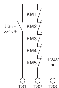
マニュアルリセットモード
