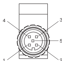
D40A-2コネクタタイプのピン配列図
