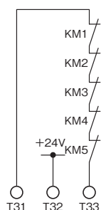
オートリセットモード
