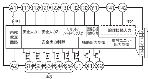
G9SX-AD322-□(高機能ユニット)
