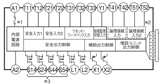
G9SX-ADA222-□(高機能ユニット)
