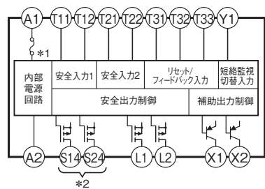
G9SX-BC202-□(単機能ユニット)
