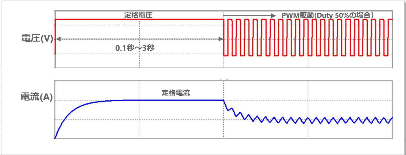
[図26:PWM制御回路におけるコイル電圧・電流波形例]
