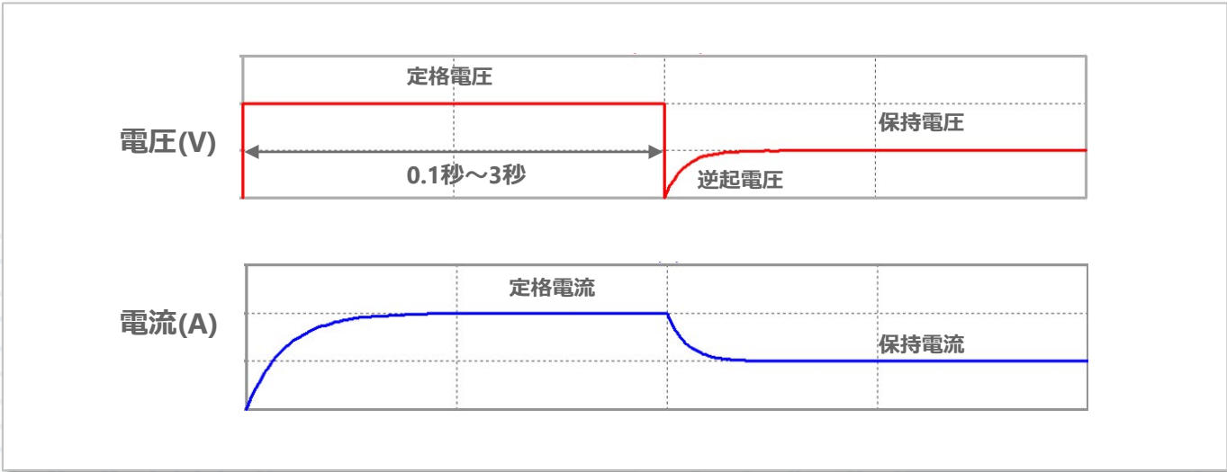
[図22:スイッチによる保持回路におけるコイル電圧・電流波形例]
