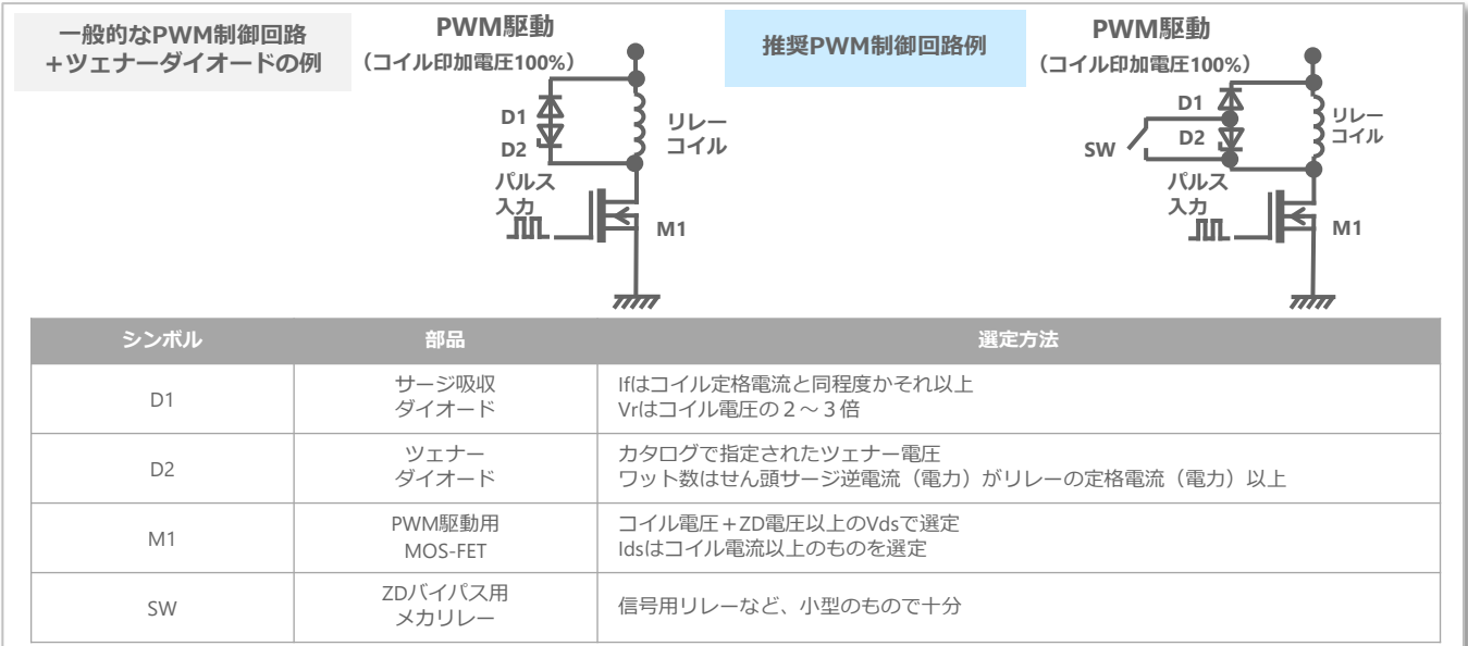
[図25:PWM制御回路例、周辺部品の選定方法]
