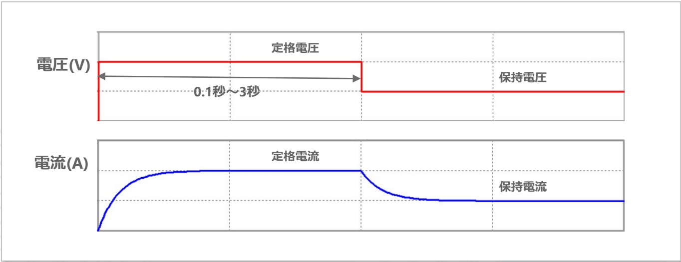
[図24:スイッチによる保持回路におけるコイル電圧・電流波形例]
