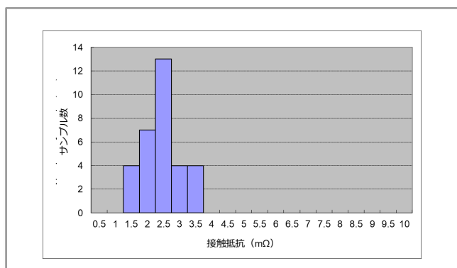
図9: G9KBシリーズの接触抵抗初期値（実測値）
