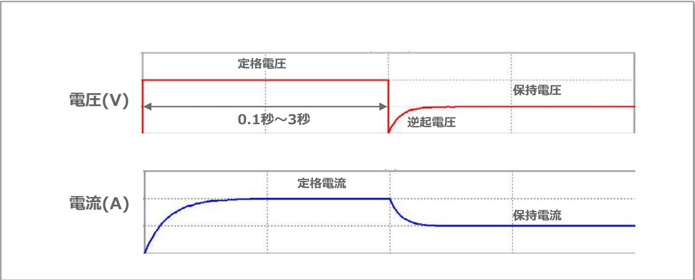
図19：スイッチによる保持回路におけるコイル電圧・電流波形例
