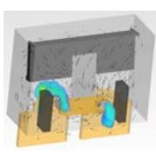
図6: アークシミュレーション技術による解析例
