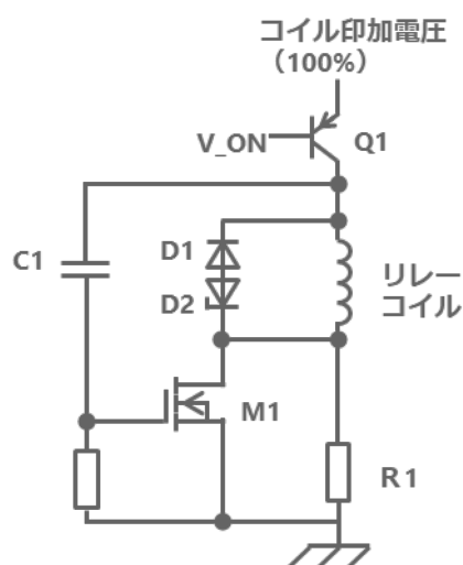
図16:保持電圧CR回路例、周辺部品の選定方法
