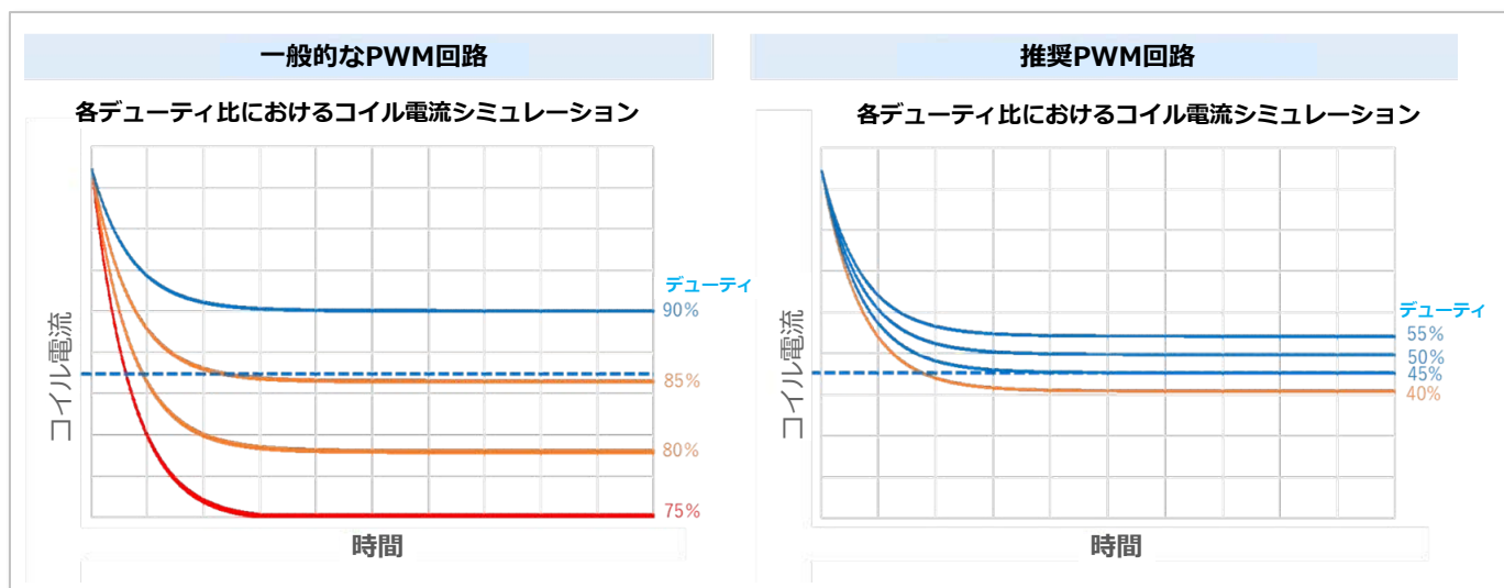
図24: PWM制御時の電流推移
