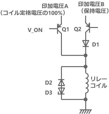
図20：スイッチによる推奨保持電圧回路例、周辺部品の選定方法
