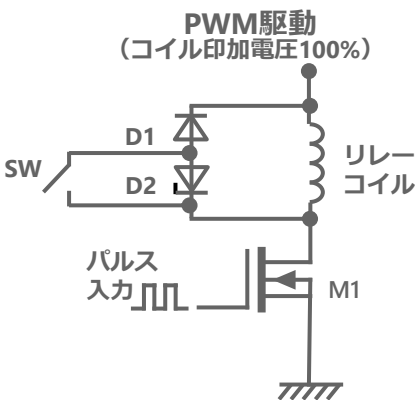
推奨PWM制御回路例
