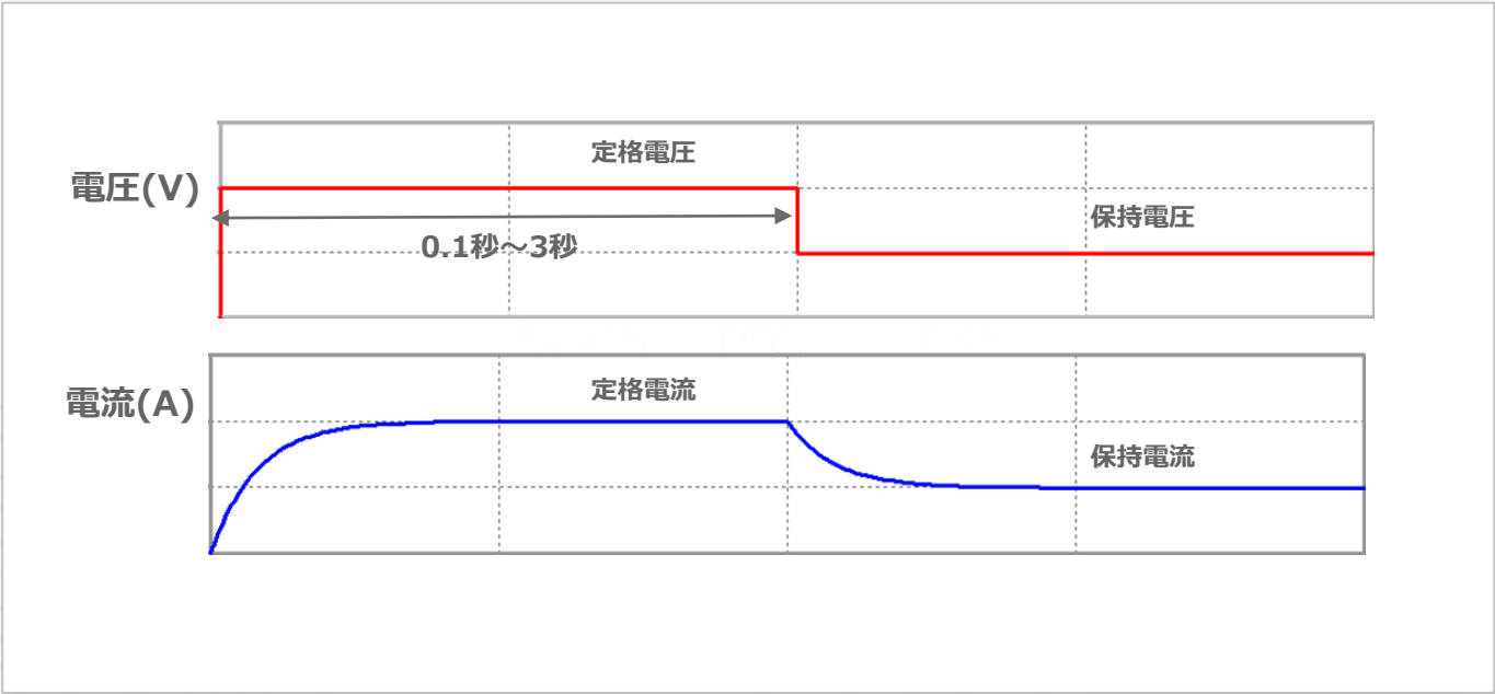
図21:スイッチによる保持回路におけるコイル電圧・電流波形例
