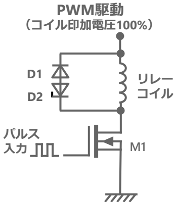
一般的なPWM制御回路 +ツェナーダイオードの例
