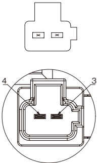
詳細図 A
