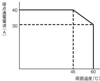
(図1) 周囲温度と接点通電電流
