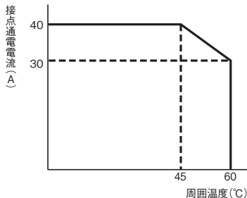
(図1) 周囲温度と接点通電電流
