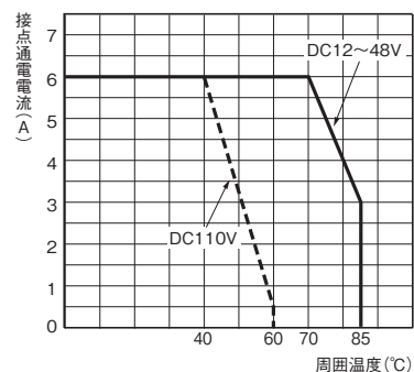
(図1) 周囲温度と接点通電電流
