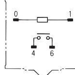
端子配置/内部接続図 (TOP VIEW)
