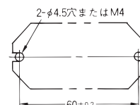
取り付け穴加工寸法
