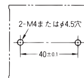
取り付け穴加工寸法
