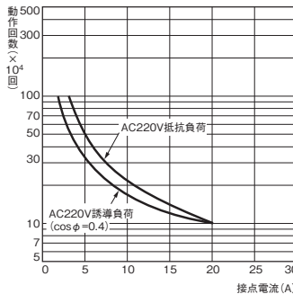
耐久性曲線
