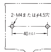
取り付け穴加工寸法
