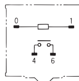
端子配置/内部接続図 (TOP VIEW)
