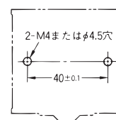
取り付け穴加工寸法
