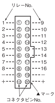
コネクタピン配置図 (TOP VIEW)
