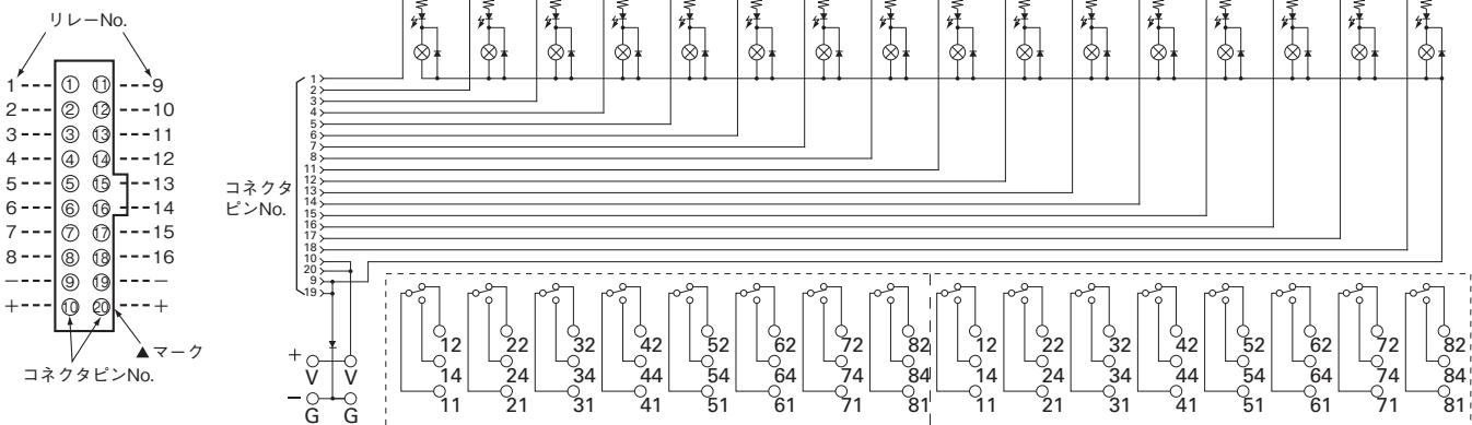
コネクタピン配置図 (TOP VIEW)
