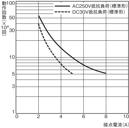
耐久性曲線
