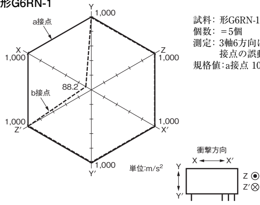
誤動作衝撃 形G6RN-1
