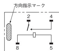
端子配置 / 内部接続図 (BOTTOM VIEW)
