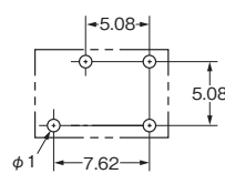
プリント基板加工寸法 (BOTTOM VIEW) 寸法公差は \pm 0.1 \text{ mm} です。
