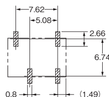
プリント基板加工寸法 (TOP VIEW) 寸法公差は \pm 0.1 \text{ mm} です。
