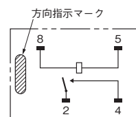
端子配置 / 内部接続図 (TOP VIEW)
