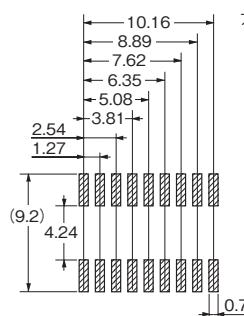
プリント基板加工寸法 (TOP VIEW) 寸法公差は±0.1mmです。
