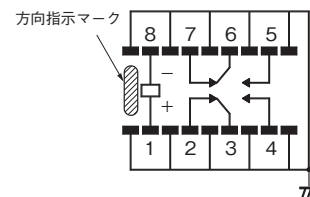
端子配置/内部接続図 (TOP VIEW)
