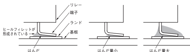
はんだ付けの良い状態
