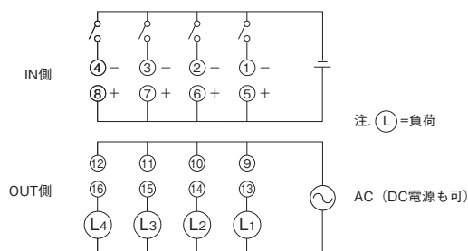
端子接続例
