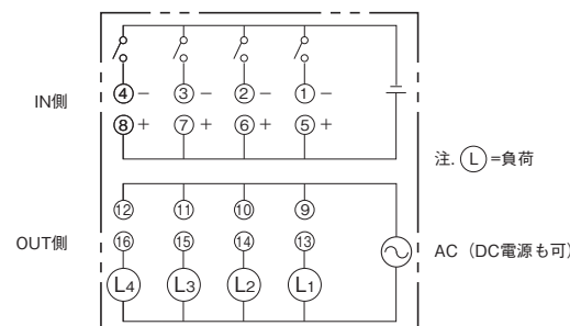
端子接続例
