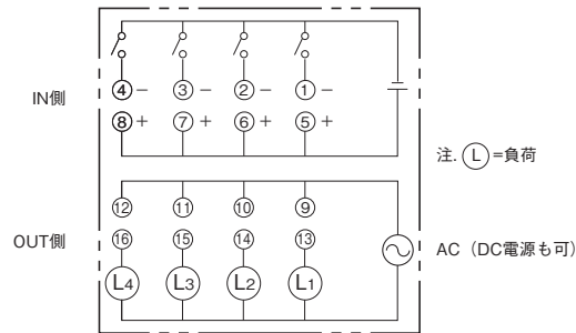
端子接続例
