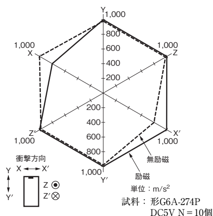
誤動作衝撃 形G6A-274P
