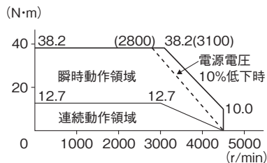
・形R88M-K4K030H/T (4kW)
