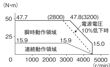
・形R88M-K5K030H/T (5kW)
