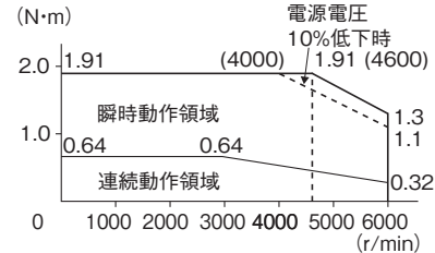
・形R88M-K20030H/T (200W)
