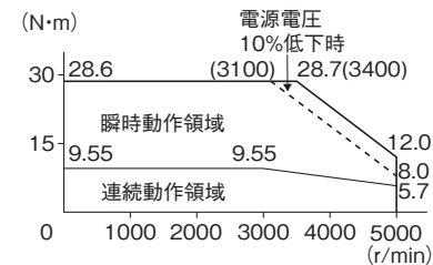
・形R88M-K3K030H/T (3kW)
