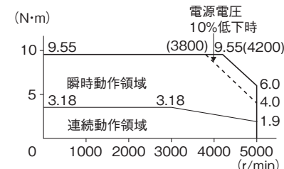
・形R88M-K1K030H/T (1kW)
