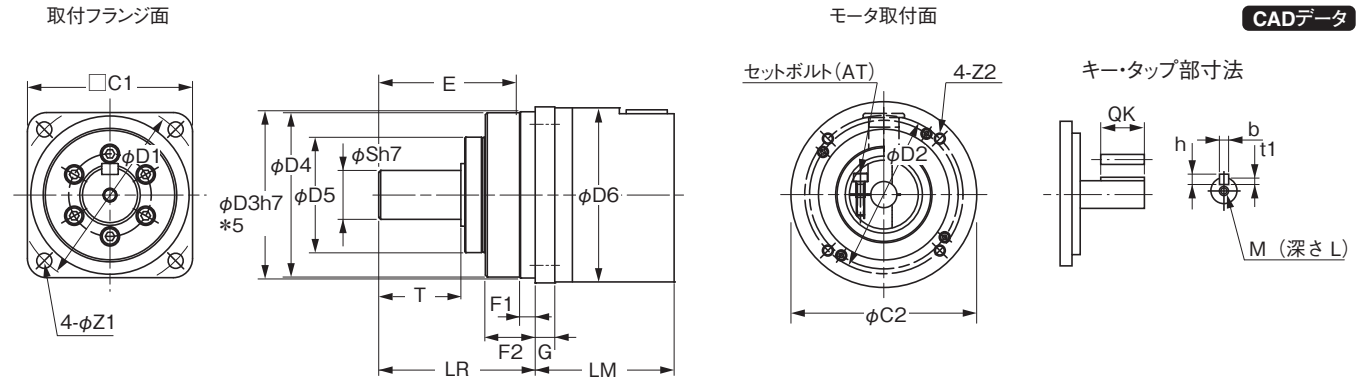
外形図2
