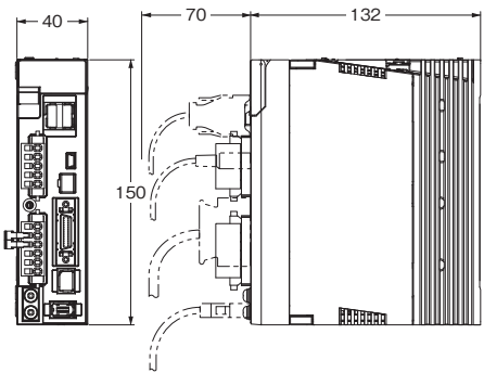
外形寸法
