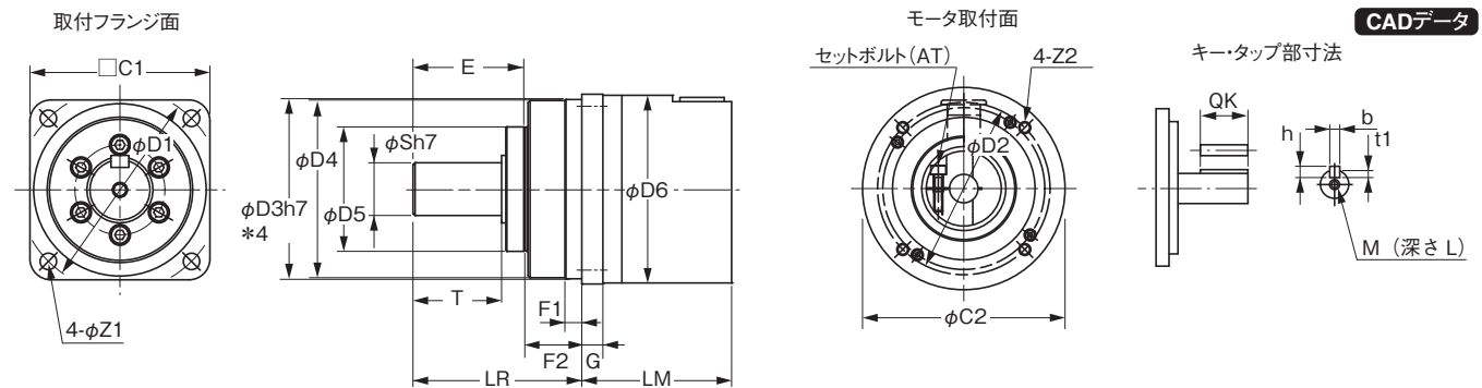
外形図2
