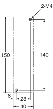
取付寸法
