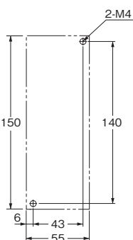
取付寸法
