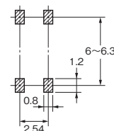
実装パッド寸法(推奨値)(TOP VIEW)
