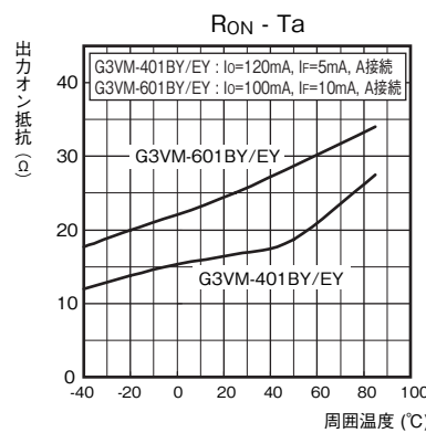
●出力オン抵抗－周囲温度
