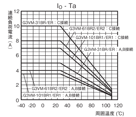
●連続負荷電流－周囲温度
