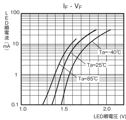
●LED順電流－LED順電圧
