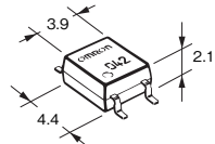
SOP4ピン
