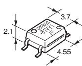
SOP4ピン特殊
