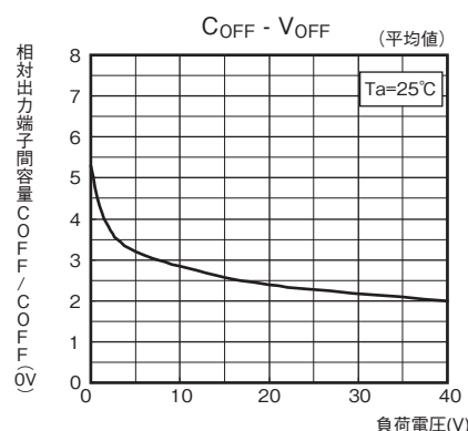
●相対出力端子間容量－負荷電圧 形G3VM-101LR
