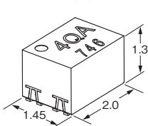
S-VSON (L) 4ピン
